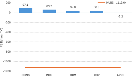
PE ratios
