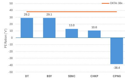
PE ratios
